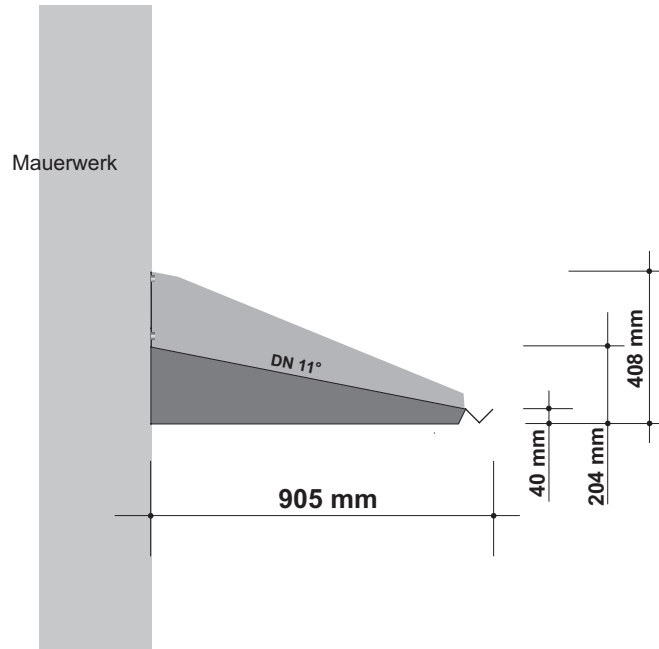
Seitenansicht
